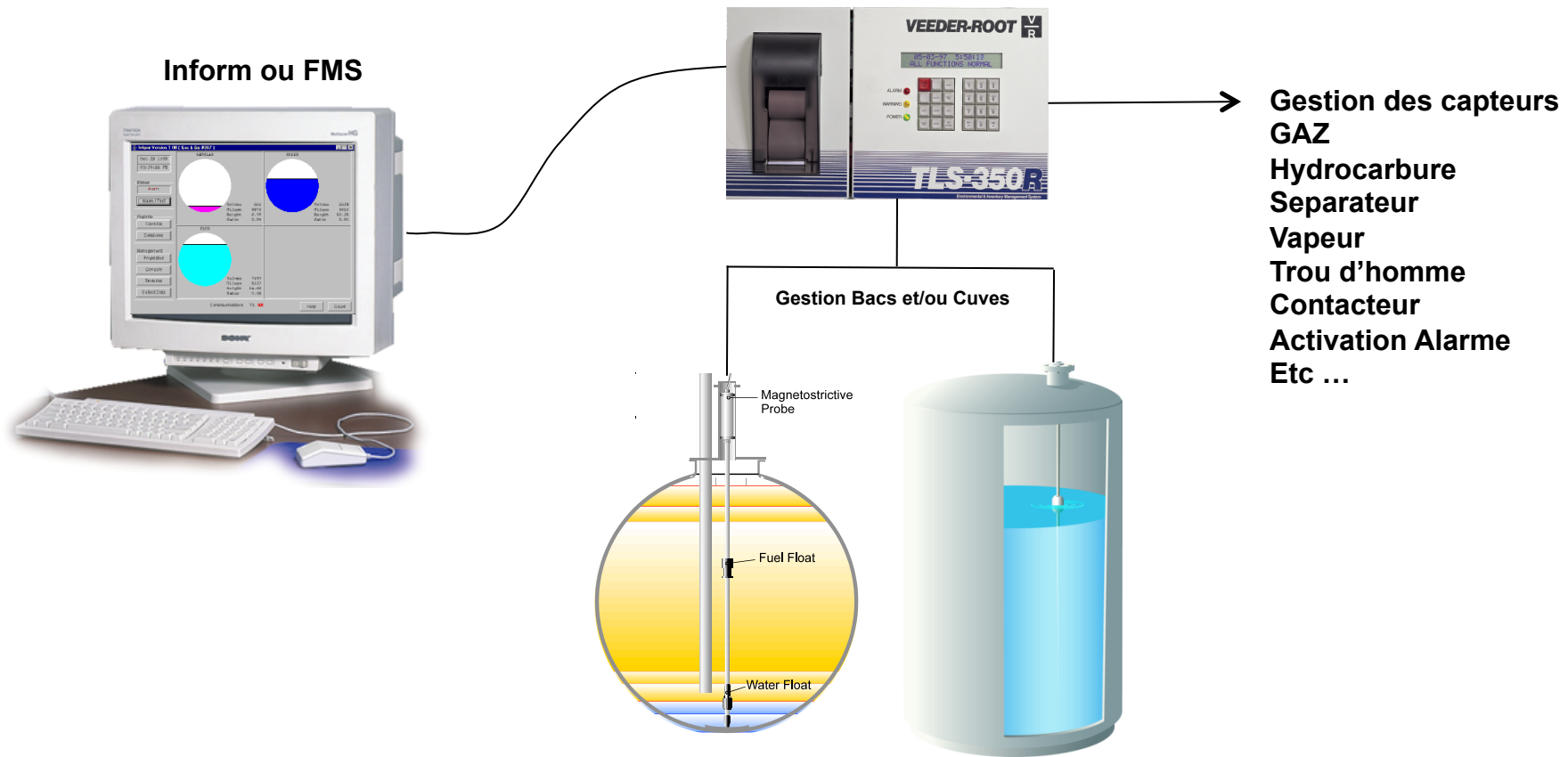
Sonde magnétostrictive Veeder-Root
